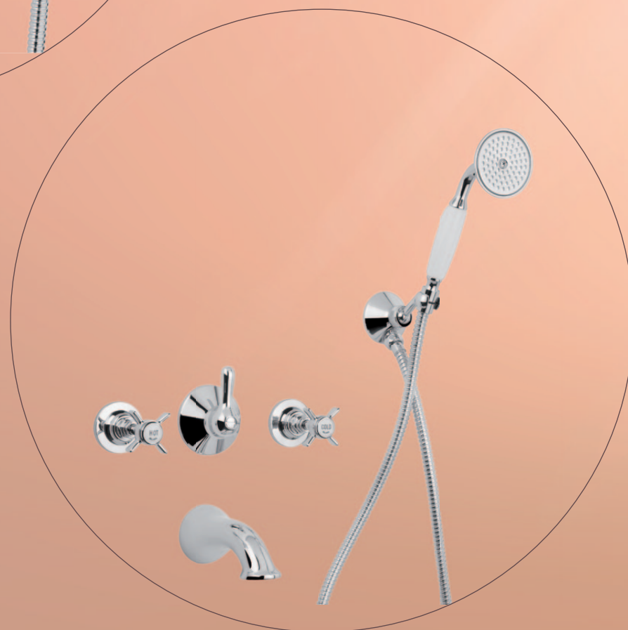
B3-116/A/E + 034133 Gruppo incasso c/deviatore 2 uscite + bocca e duplex completo Built-in group with diverter 2 outputs + spout and complete duplex встраиваемого смесителя с переключателем на 2 выхода + излив и душевой набор
